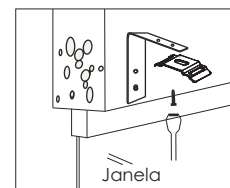
Parede
